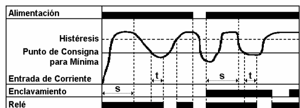
SP-104: Detección por Mínima o Infracarga
