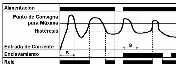
SP-101: Detección por Máxima o Sobrecarga
