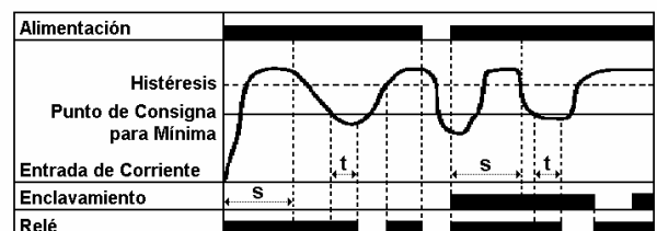
SP-103: Detección por Mínima o Infracarga
