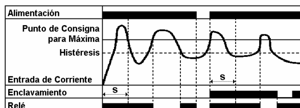
SP-100: Detección por Máxima o Sobrecarga
