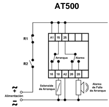
Cableado Típico
